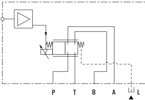
Typ KBTG4V-5 Proportional-Drosselventil (mit integrierter Elektronik)
